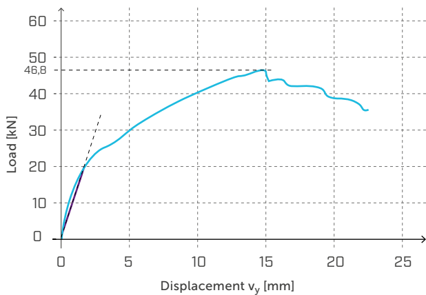
Kraft-Verschiebung-Diagramme für TCP300-Probe mit teilweiser Ausnagelung (Nr. 14 LBA-Nägel Ø4 x 60 mm).
