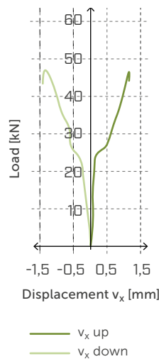
Kraft-Verschiebung-Diagramme für TCP300-Probe mit teilweiser Ausnagelung (Nr. 14 LBA-Nägel Ø4 x 60 mm).
